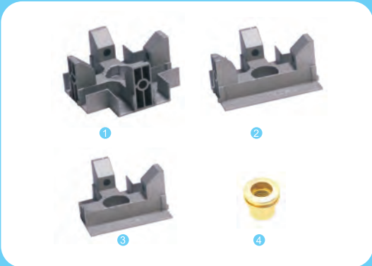
1. 槽液型: JH008D四通 2. 槽液型: JH008D三通 3. 槽液型: JH008D二通 4. M5拉姆
