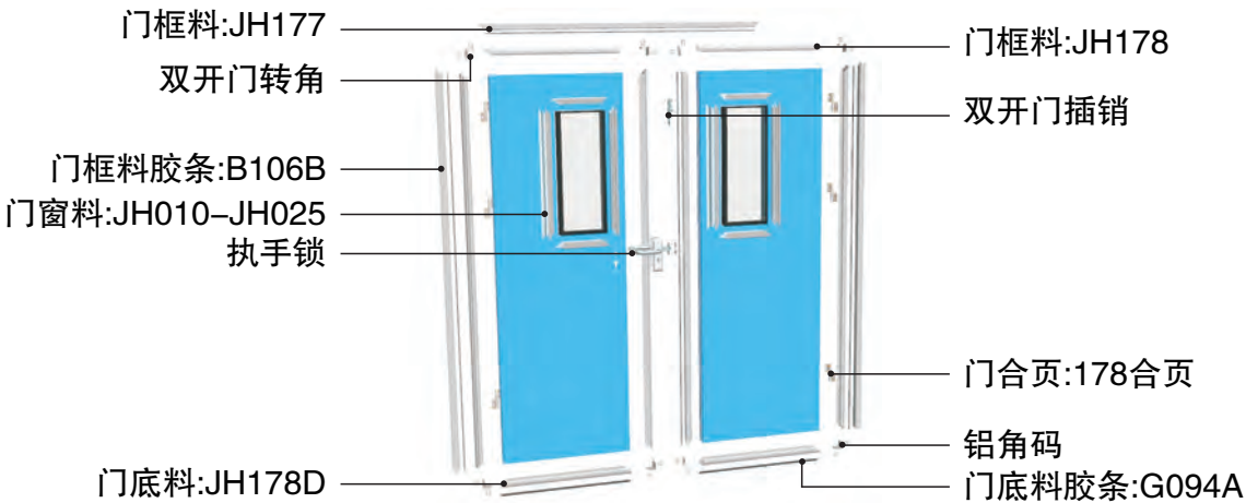
JH178D双开门分解图
